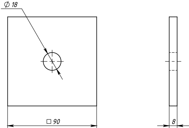
Поз.3 (Плита)
